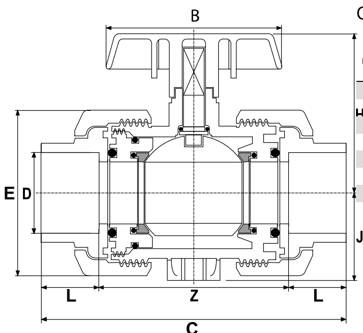
Válvula esfera encolar
