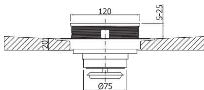
Sección desagüe vertical
