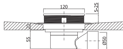
Sección desagüe horizontal
