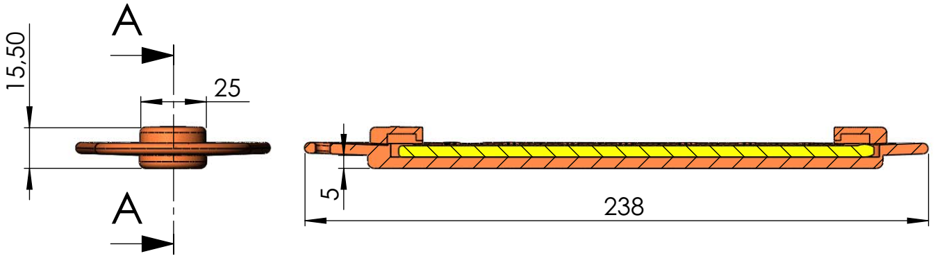
SECCIÓN A-A
