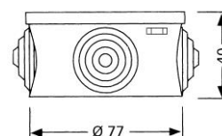
Ref. 665 4 conos para tubo de Ø 20 (M20).
