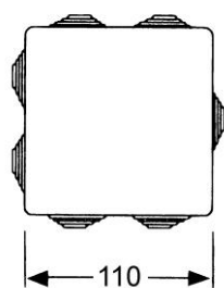
Ref. 615 7 conos para tubo de Ø 25 (M25).
