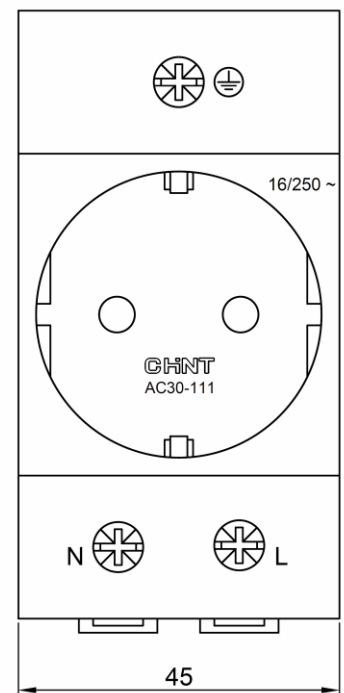
Dimensiones (medidas en mm)
